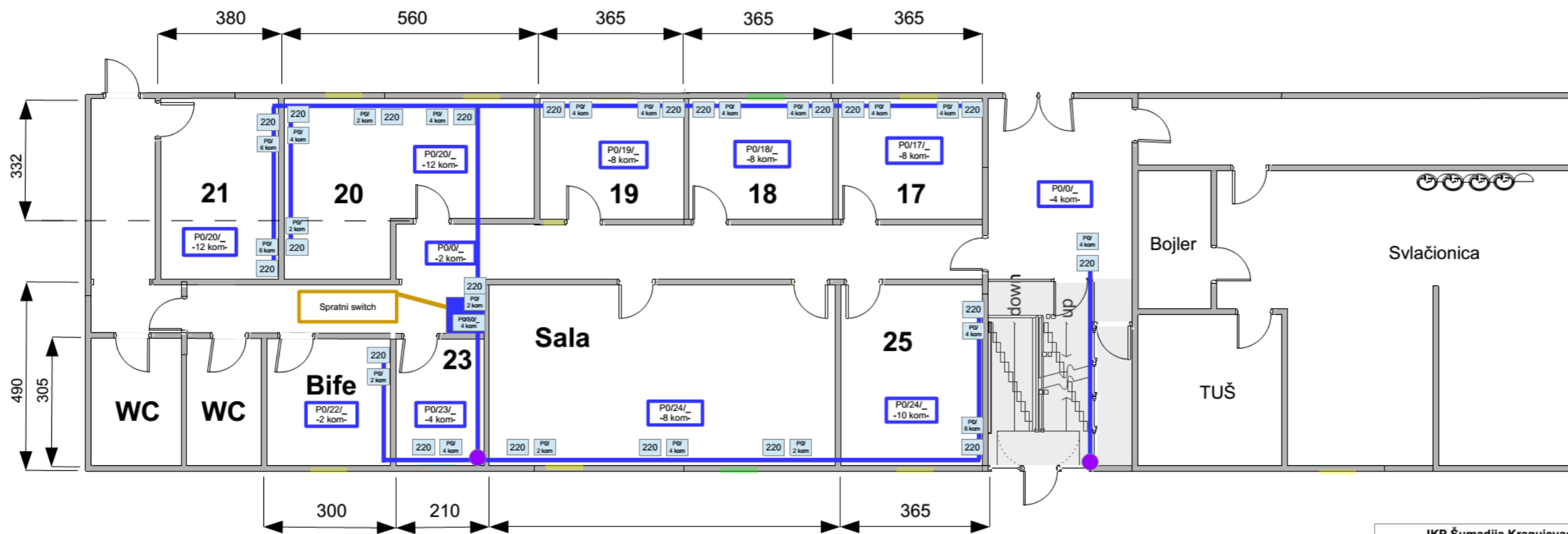
Шема 1 – предлог мрежног развода
